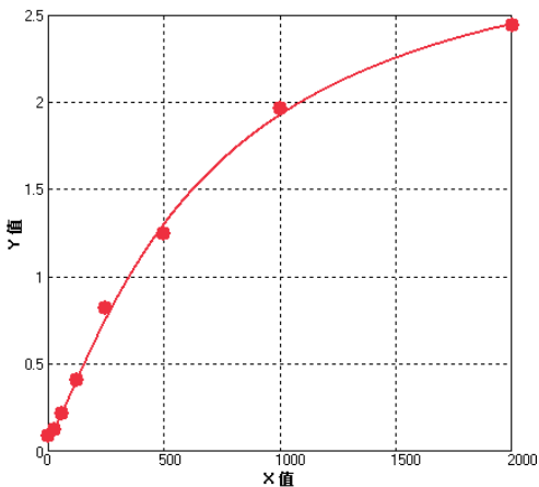
人CCL17参考标准曲线
