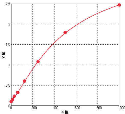
人PTH参考标准曲线
