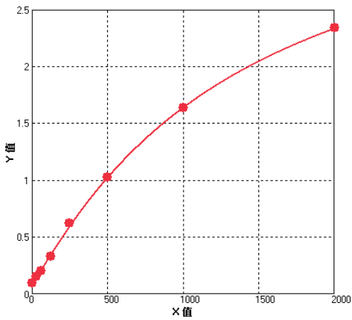
人CCL24参考标准曲线
