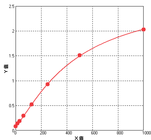
人IL-4R参考标准曲线
