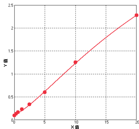
人CD26参考标准曲线
