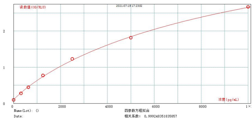
人 CRP 参考标准曲线(超敏)
