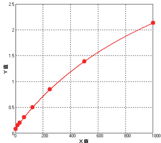
小鼠IL-10参考标准曲线
